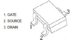
SOT-523
